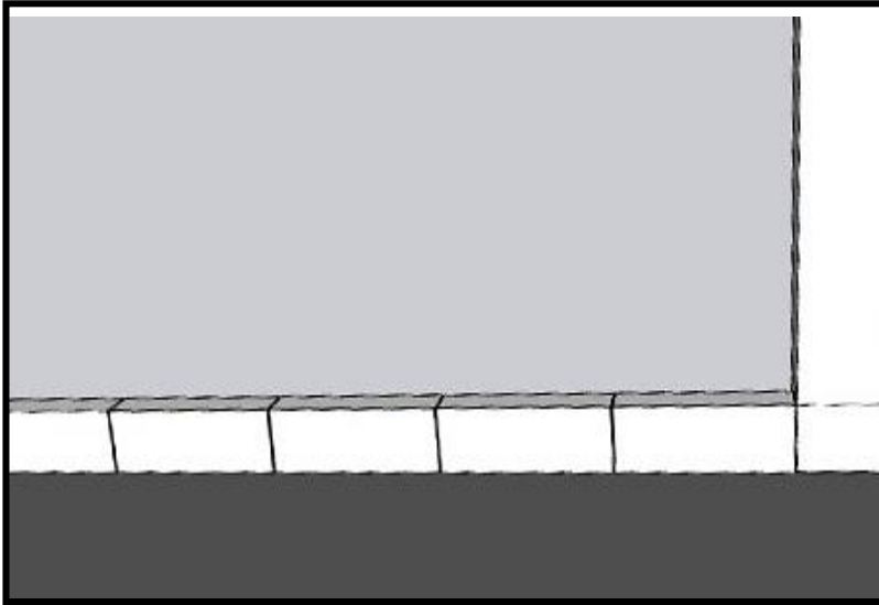
ধাপ ৪: প্রস্তুতকৃত মর্টারের স্তরের ওপর একটি করে ব্লক স্থাপন করতে হবে। একই মর্টার দিয়ে ব্লকগুলোর মধ্যে জয়েন্টগুলো পূরণ করতে হবে। একটি স্তরের ব্লক বসানো সম্পন্ন হলে পরবর্তী স্তরের ব্লক বসানোর কাজ শুরু করতে হবে।
