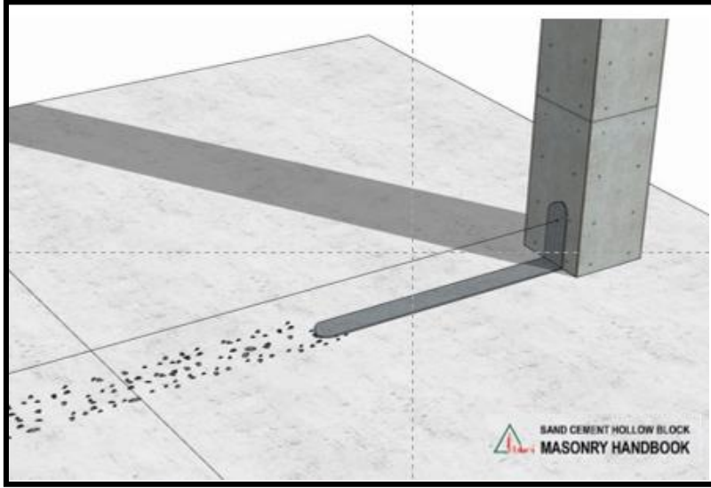
ধাপ ৩: ব্লক স্থাপনের তল সমতল করার জন্য প্রথমে মর্টারের একটি স্তর (সিমেন্ট: বালি- ১:৪) দিতে হবে।
